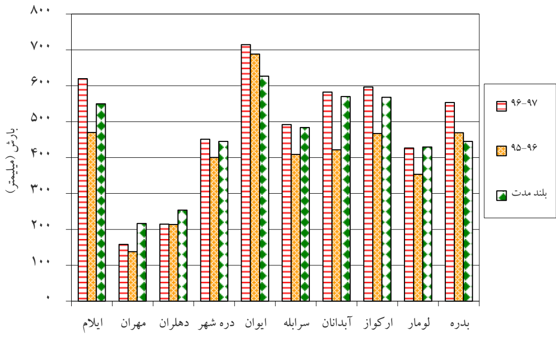
آمار بارندگی مراکز شهرستانهای استان ایلام از اول مهرماه ۹۶ لغایت ۲۳ اردیبهشت ماه ۹۷ و مشابه آن در سال ۹۵-۹۶ و بلند مدت (دوره آماری موجود)
